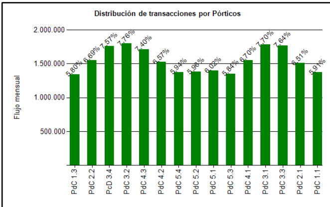
Gráfico 3: Distribución de Flujos por Pórtico de Cobro, Abril 2015. Fuente: Reporte 29 SICE.
